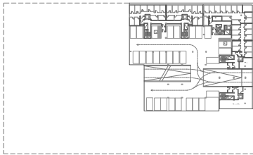
NIVEL -1
