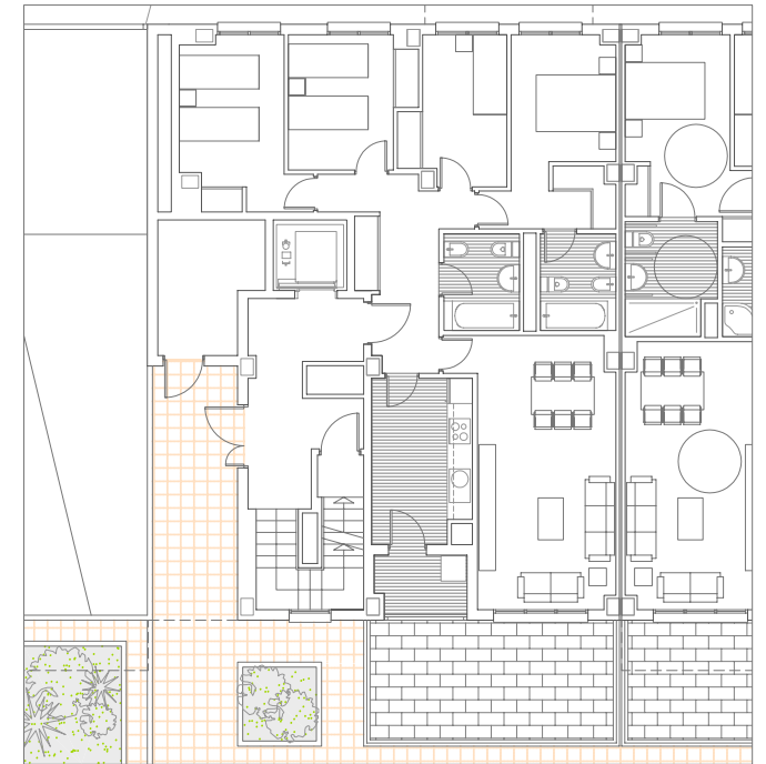
TIPOLOGIA 4D1
