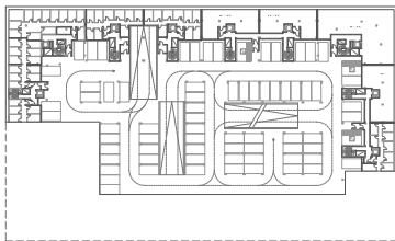
NIVEL -2
