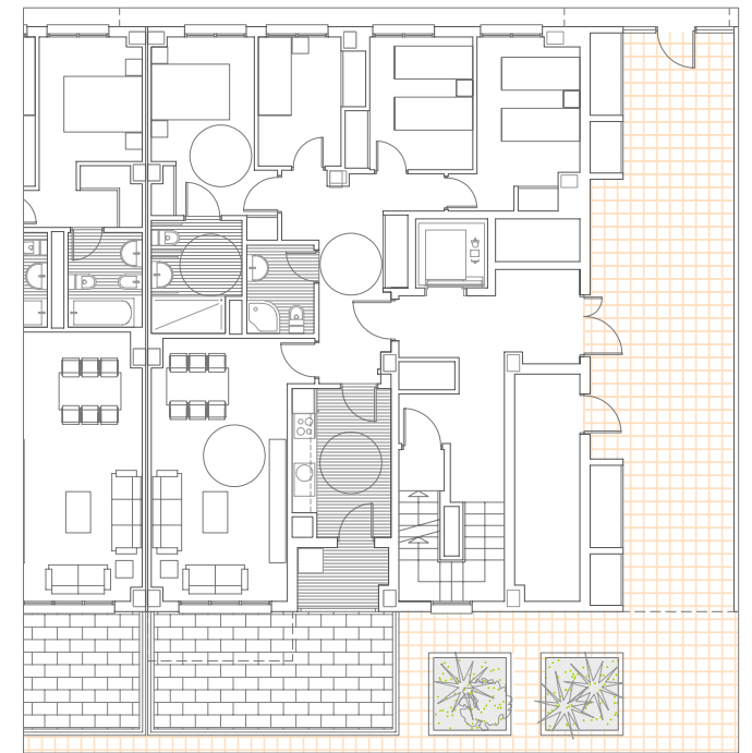
TIPOLOGIA 4D2M
