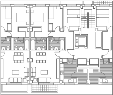
TIPOLOGIA 3D7
